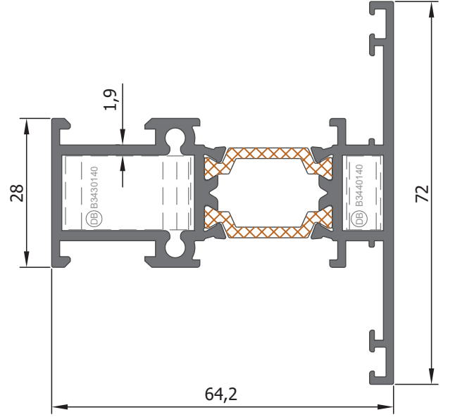
Orta Kayıt Profili 1.9 mm. Transom Profile
