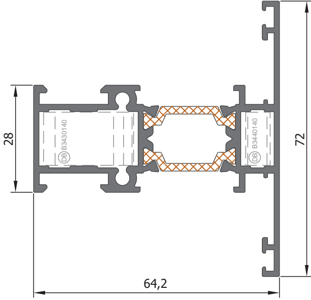
Orta Kayıt Profili 1.4 mm. Transom Profile
